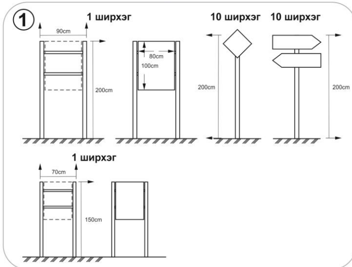
Зураг-8: Самбар, анхаруулах тэмдэг, зүг заасан тэмдэгийн төлөвлөлт
