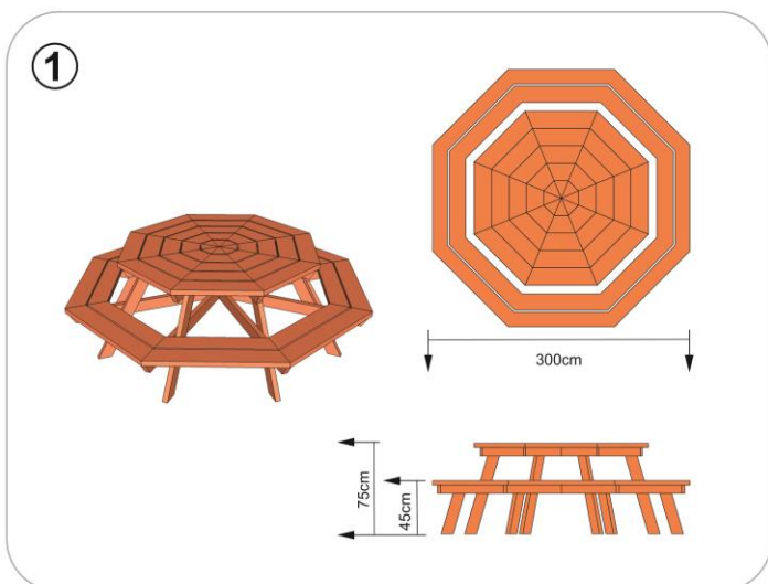
Зураг-7: 8 талт сандлын төлөвлөлт
